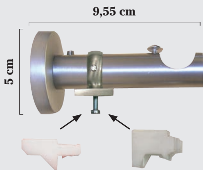
Soporte con Adaptador de Riel
